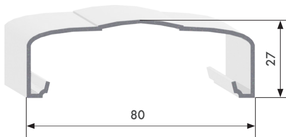
COUPE DU CAPOT DE BARRE
