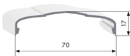
CADRE DE RÉNOVATION AVEC RECOUVREMENT INTÉRIEUR
