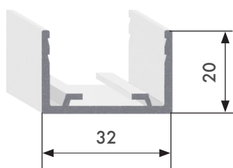
CADRE OUVRANT
