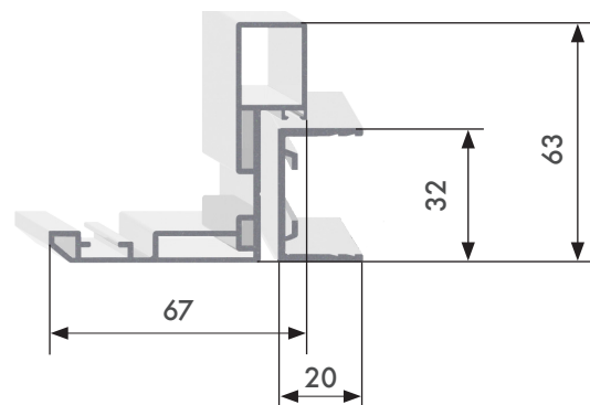
CADRE DE RÉNOVATION AVEC RECOUVREMENT INTÉRIEUR
