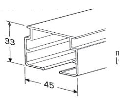
Coupe du rail anodisé marron
