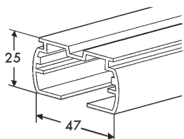
Coupe du rail laqué blanc
