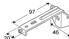
Équerre non réglable pour lame de 89 mm
