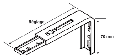
Équerre pose de face réglable
