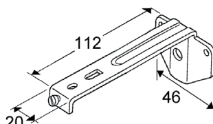
Équerre non réglable pour lame de 127 mm
